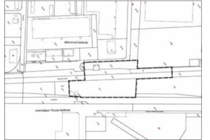
Lageplan: Geltungsbereich des Bebauungsplans Nr. 1/2023 „Verkehrsanschluss Mönchhof / Ehemaliges Ticona-Gelände“
